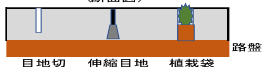
(断面図)
